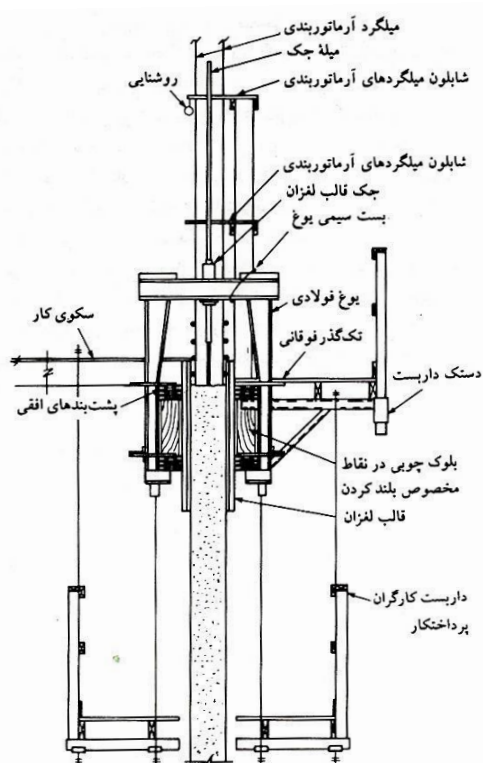
شکل ت ۵-۹ اجزای قالب لغزان
