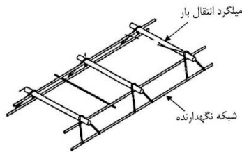
شکل ت ۱۰-۵ سبد میلگردهای انتقال بار
