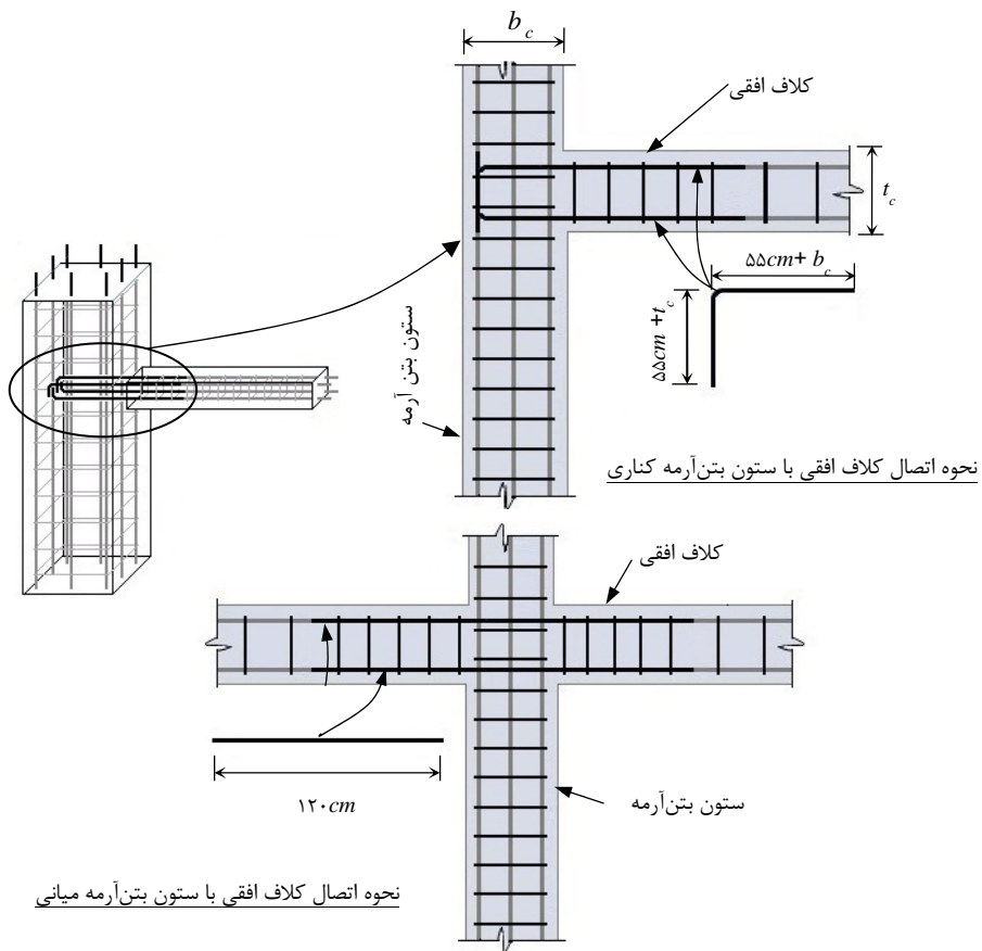
شکل ۷-۱۹ جزئیات میلگردگذاری برای اتصال کلاف افقی به سستون بتن آرمه
